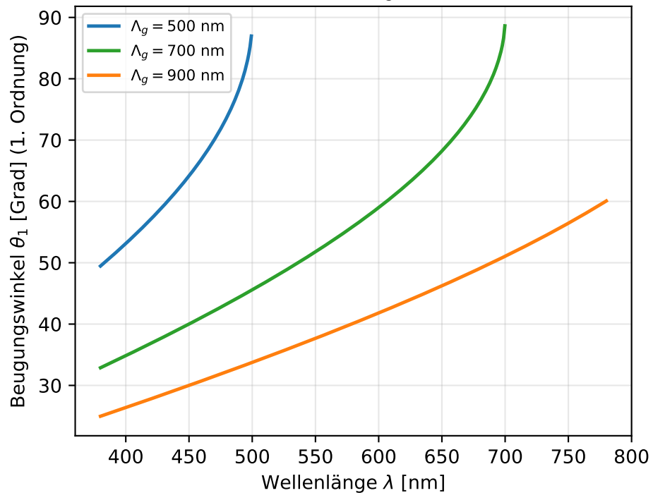
Gittergleichung: \Lambda_g \sin \theta_m = m\lambda
