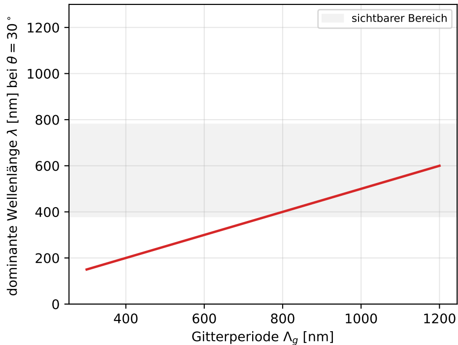
Periodenabhängigkeit der Beugungsfarbe
