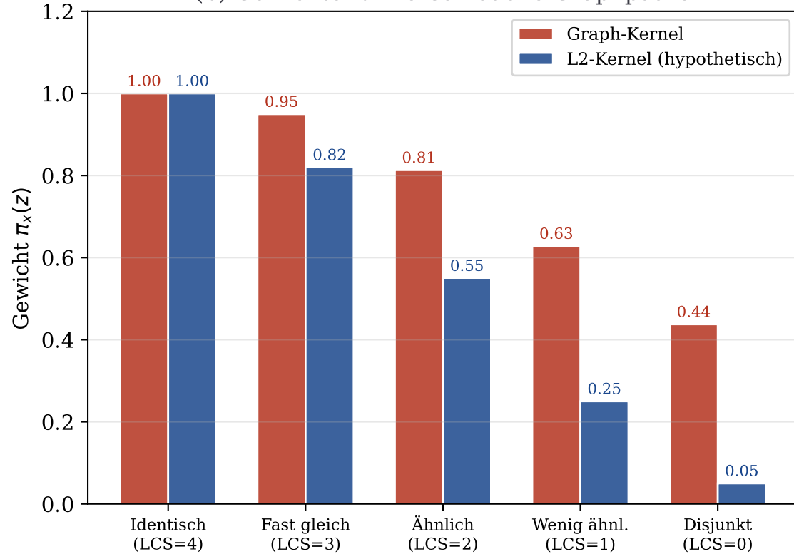
(b) Gewichte für verschiedene Graphpaare
