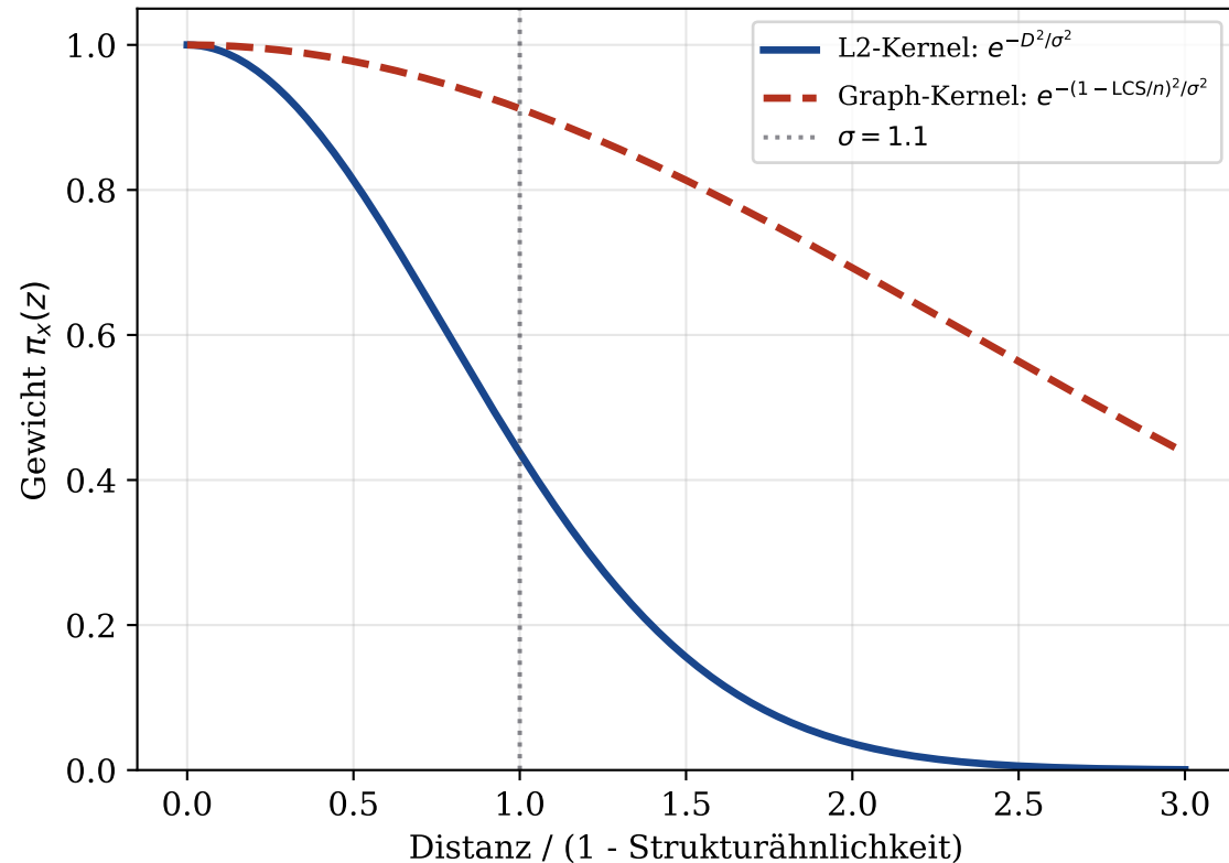
(a) Vergleich der Kernelfunktionen
