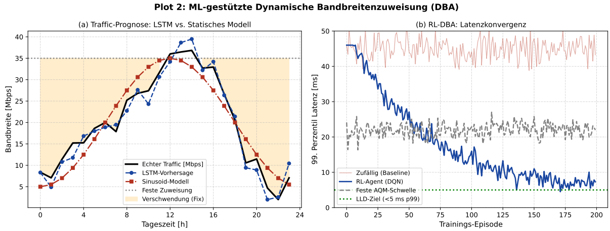
Figure 2: ML-gestützte DBA. (a) Tages-Traffic-Prognose: LSTM-Modell (blau, gestrichelt) approximiert den echten Traffic (schwarz) wesentlich genauer als das sinusoidale Basismodell (rot), insbesondere bei unerwarteten Lastspitzen. Die orange Fläche zeigt die Verschwendung bei fixer Zuweisung (grau gepunktet). (b) RL-DBA-Latenzkonvergenz über Trainings-Episoden: Der DQN-Agent (blau) lernt, die p99-Latenz von initial über 40 ms auf unter 5 ms (grüne LLD-Grenze) zu reduzieren, während die feste AQM-Schwelle (grau) dauerhaft über dem Ziel verbleibt.
