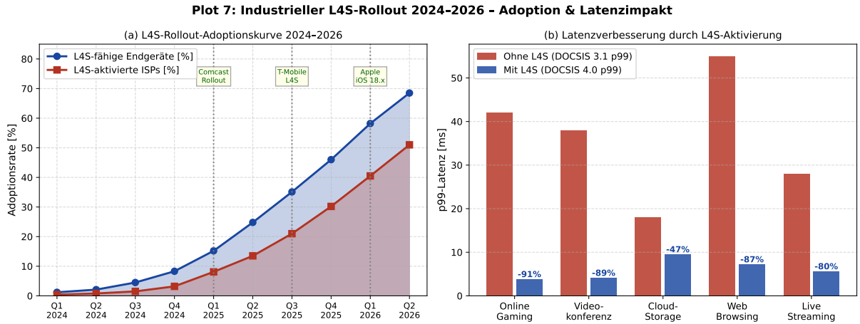
Figure 7: Industrieller L4S-Rollout 2024–2026. (a) Adoptionskurven für L4S-fähige Endgeräte (blau) und ISPs (rot) von Q1-2024 bis Q2-2026. Markierte Ereignisse: Comcast-Rollout (Q1-2025), T-Mobile-L4S-Ankündigung (Q3-2025), Apple iOS 18.x-Integration (Q1-2026). Die kritische Adoptiosschwelle \eta^* = 0.5 wurde in Q2-2026 überschritten. (b) Latenzverbesserung pro Anwendungsfall durch L4S-Aktivierung: Online-Gaming profitiert mit -91\% am stärksten; auch Videokonferenz ( -89\% ) und Web-Browsing ( -87\% ) zeigen dramatische Verbesserungen.
