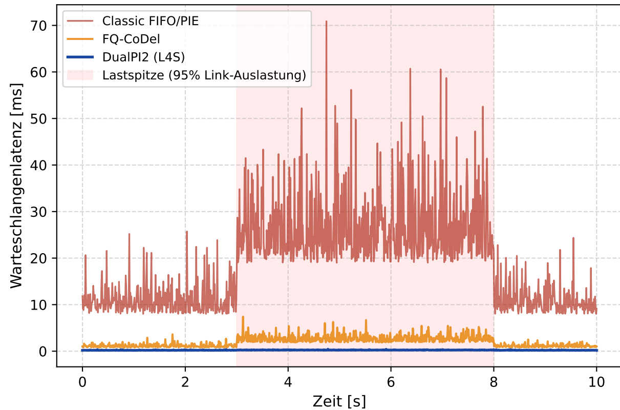
(a) Latenzvergleich: Classic vs. L4S AQM
