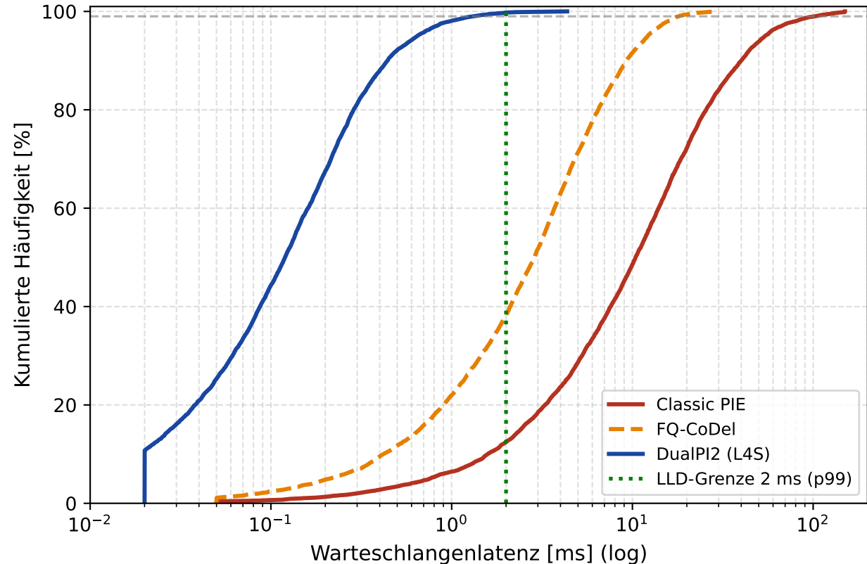
(b) CDF der Warteschlangenlatenz
