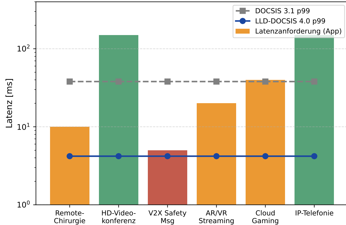
(a) App-Latenzanforderungen vs. DOCSIS-Kapazitäten
