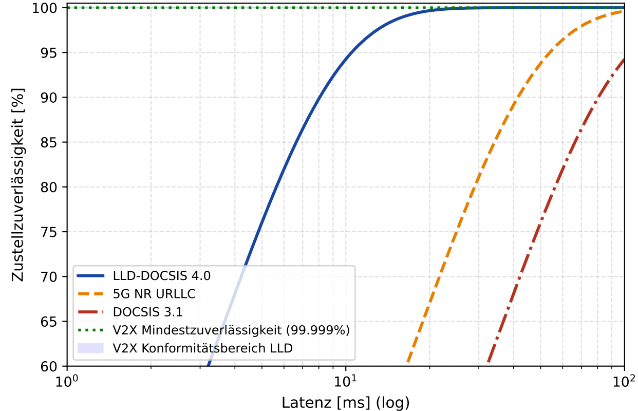
(b) Zuverlässigkeit vs. Latenz für V2X Safety
