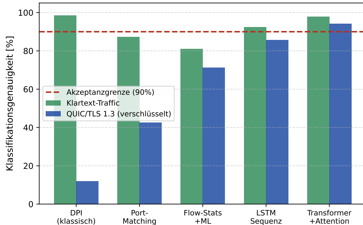
(a) Traffic-Klassifikation: Klartext vs. Verschlüsselt
