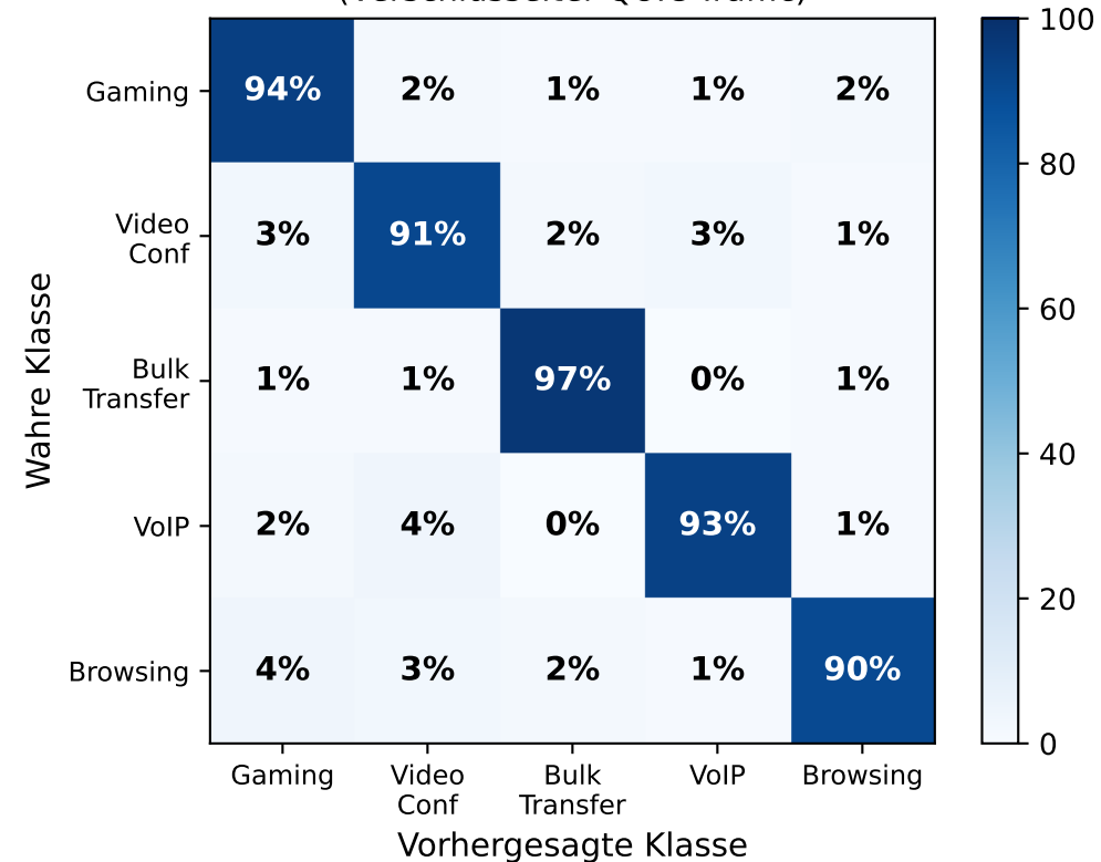
(b) Konfusionsmatrix: Transformer-Klassifikator (Verschlüsselter QUIC-Traffic)
