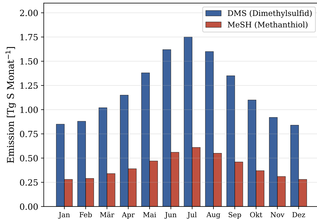
Globale marine Schwefelgas-Emissionen nach Monat
