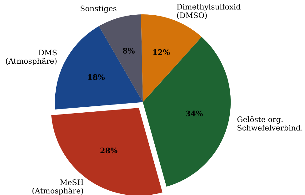
DMSP-Routing im marinen Schwefelzyklus (%-Anteile)
