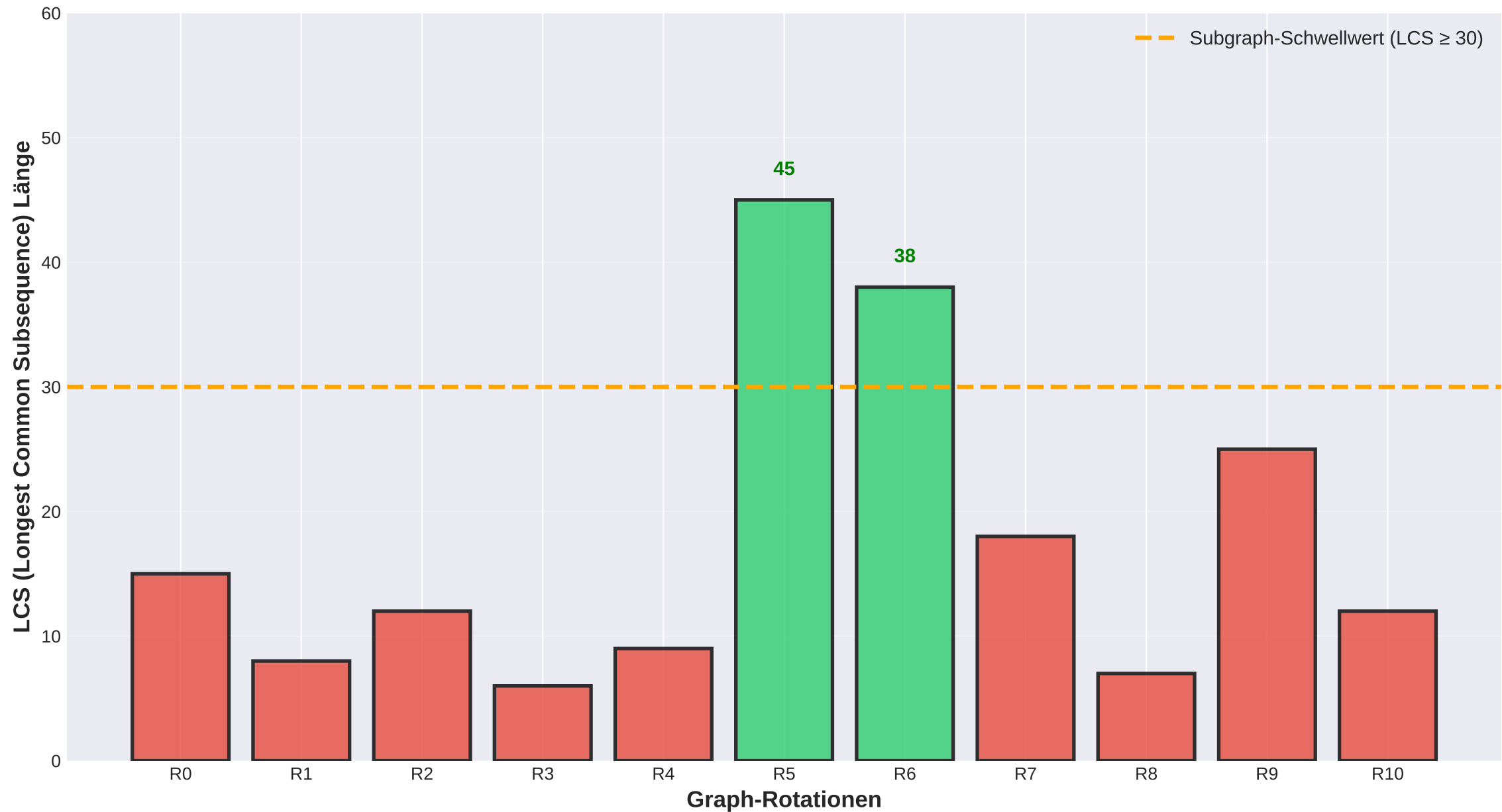
Subgraph-Matching: LCS-Scores für VP1-Sequenz-Graph vs. Struktur-Kontakt-Graph
