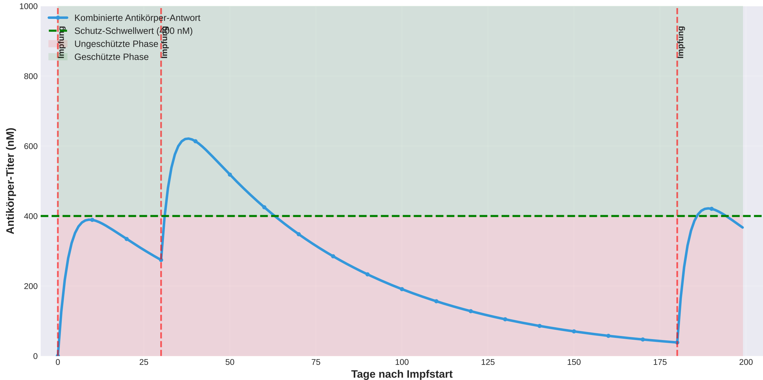
Modellierte Antikörper-Dynamik: Impfschema 0, 1, 6 Monate
