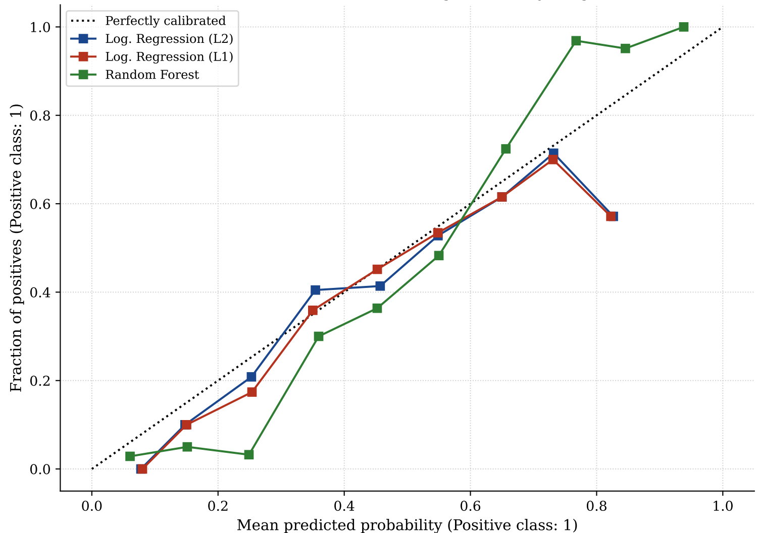
Wahrscheinlichkeitskalibrierung (Reliability Diagram)
