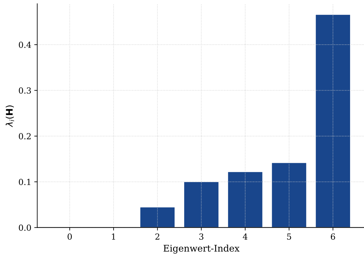
Eigenwerte der Hesse-Matrix (alle \geq 0 \Rightarrow Konvexität)
