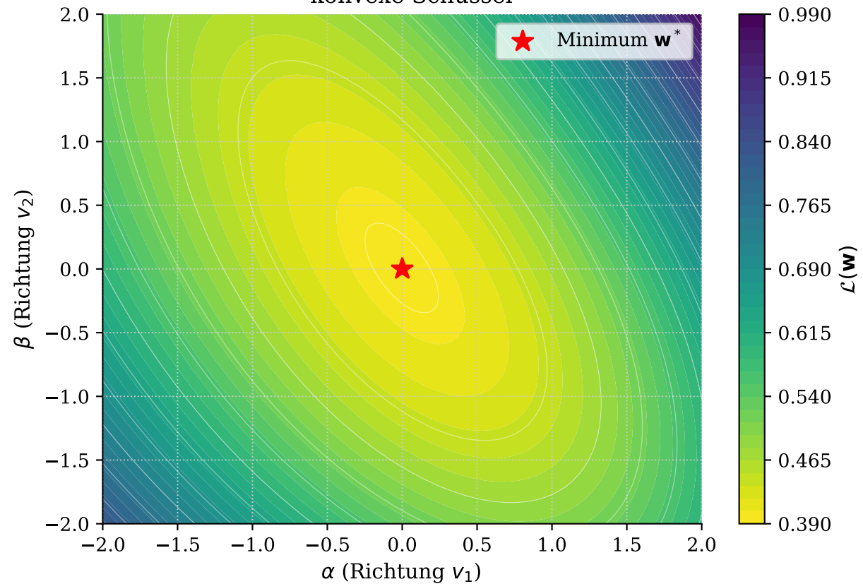
Verlustlandschaft (2D-Schnitt) - konvexe Schüssel
