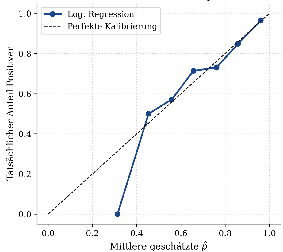
Kalibrierungsdiagramm (klinische Anwendung)
