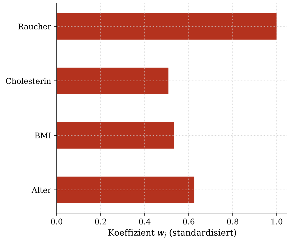
Logistische Regression: Klinische Risikofaktoren
