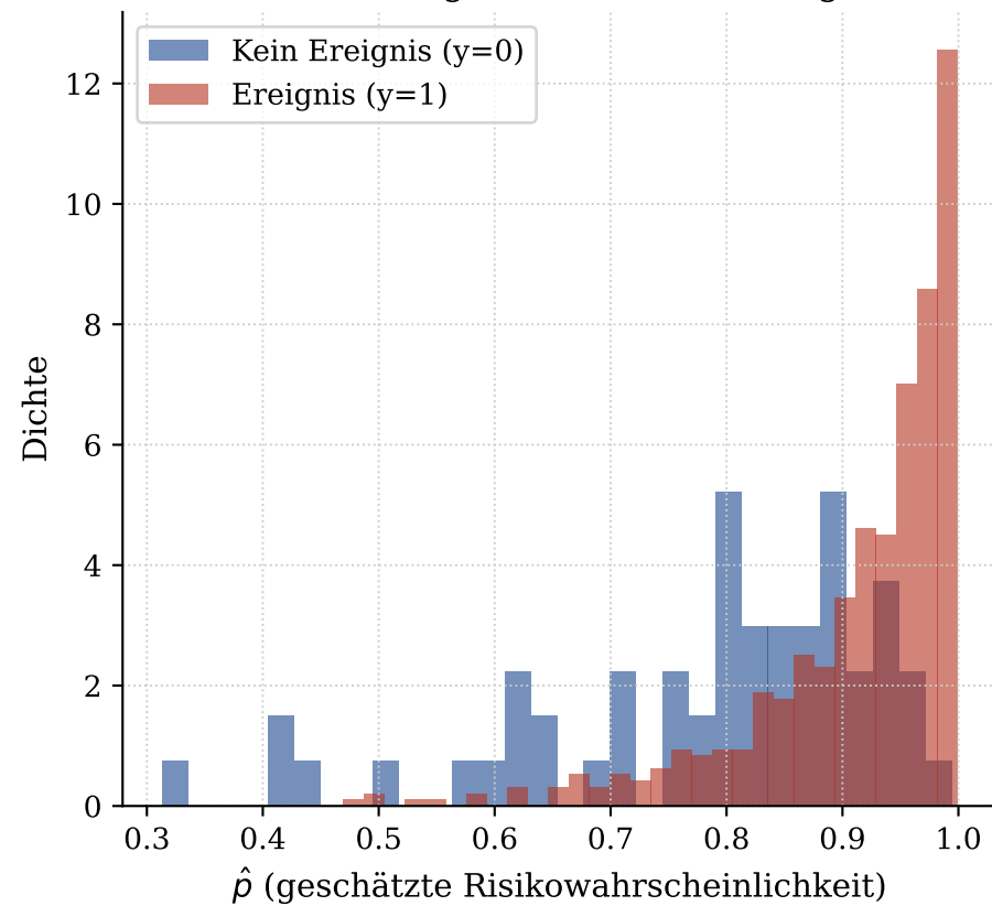
Verteilung der Risikoschätzung
