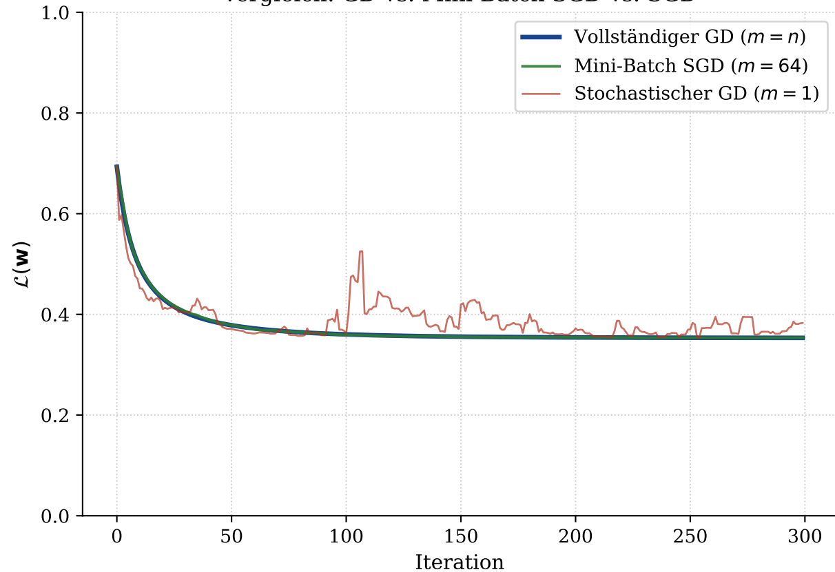
Vergleich: GD vs. Mini-Batch SGD vs. SGD
