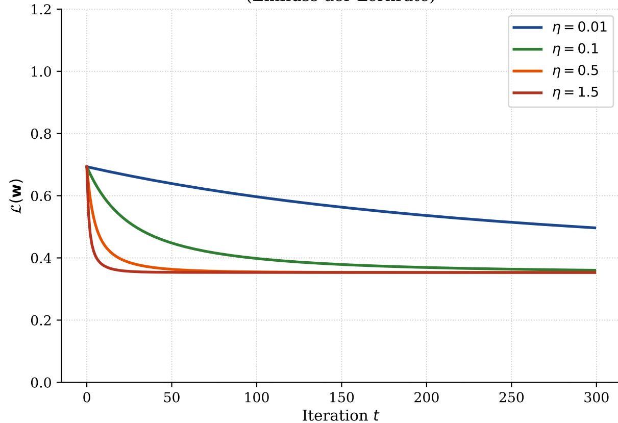
Konvergenz des Gradientenabstiegs (Einfluss der Lernrate)
