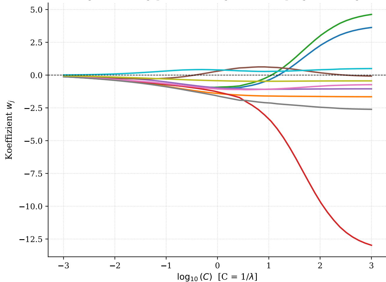
Regularisierungspfad - L2 (Ridge) - schrumpft gleichmäßig
