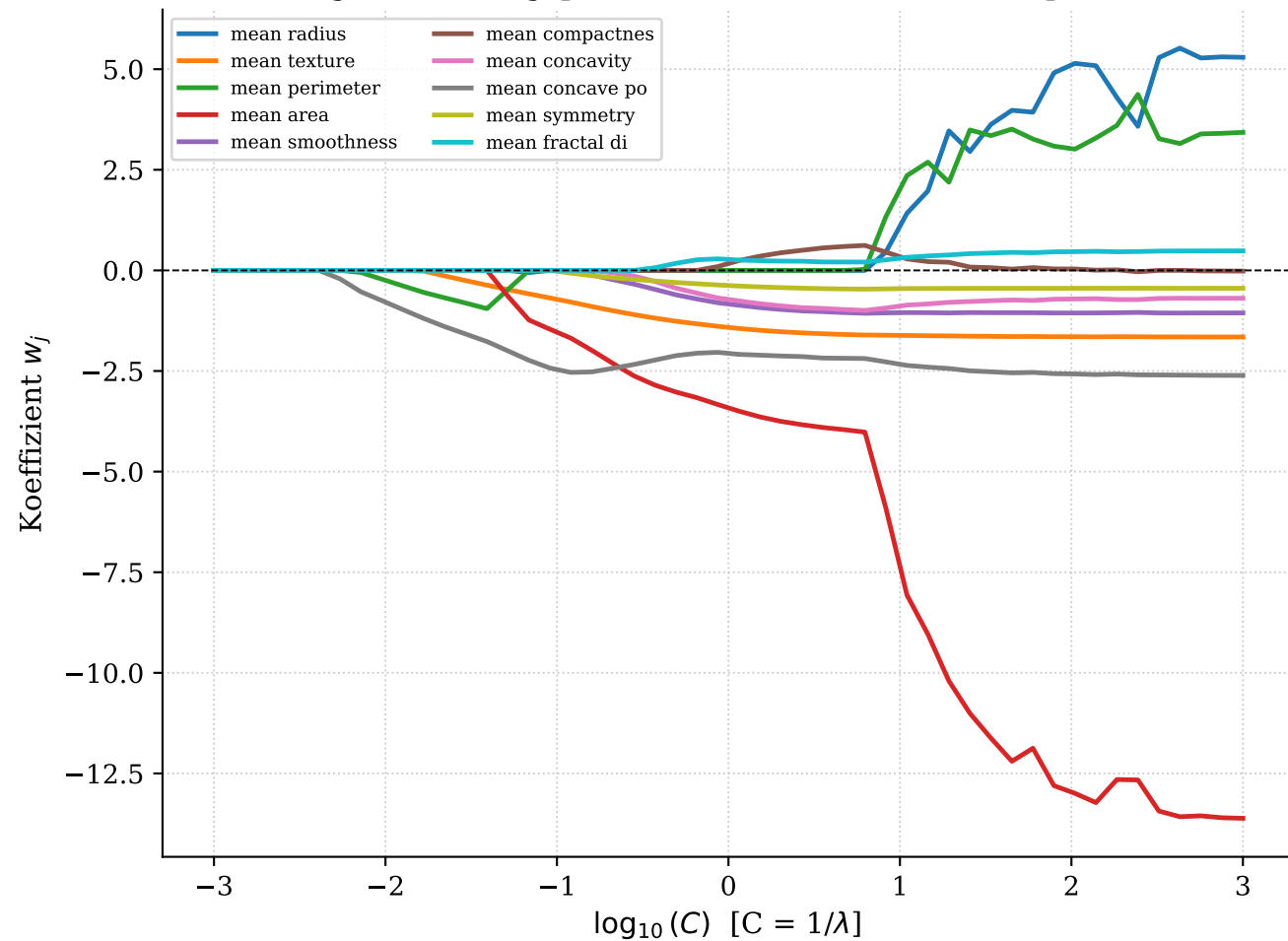
Regularisierungspfad - L1 (Lasso) - induziert Sparsität
