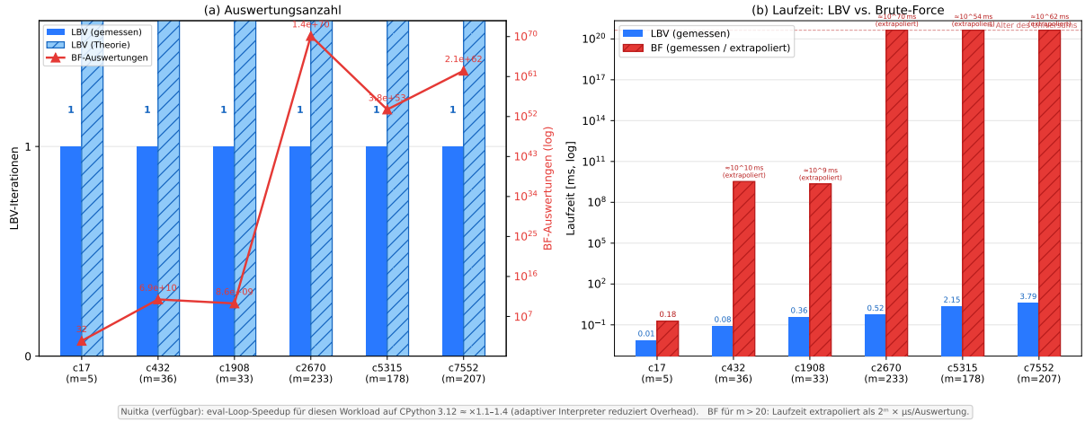
Abbildung 3: Experiment 3: ISCAS’85-Benchmarks c17, c432, c1908, c2670, c5315, c7552. (a) Auswertungsanzahl (logarithmische rechte y-Achse für BF): LBV-Iterationen gemessen (blau) und theoretische Obergrenze \lceil \log_2 m \rceil + 2 (blau schraffiert) vs. BF-Auswertungen (rot, für alle Circuits außer c17 theoretisch extrapoliert). Das LBV terminiert für alle Circuits already in Runde 1, da die Allein-Eins-Belegung die Schaltkreisausgabe erfüllt. (b) Laufzeit: LBV (gemessen) vs. Brute-Force (gemessen / extrapoliert), logarithmische y-Achse: LBV löst alle Circuits in 0,013–2,5 ms; die extrapolierte BF-Laufzeit übersteigt für Circuits ab c432 zig Tage bis hin zum Vielfachen des Weltalters – die gestrichelte horizontale Linie markiert das Alter des Universums ( \approx 4,35 \times 10^{20} ms).
