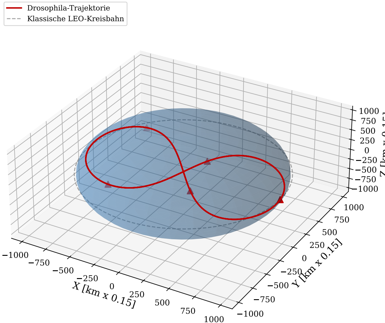
Abbildung 1: Drosophila-Lemniskaten-Trajektorie vs. klassische LEO-Kreisbahn ( h = 100 km)
