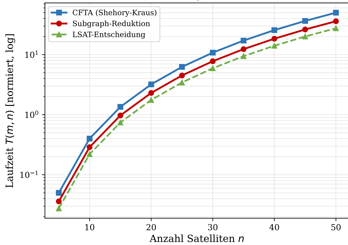
Abb. 3b: Laufzeitvergleich ( m = 20, k = 3 )
