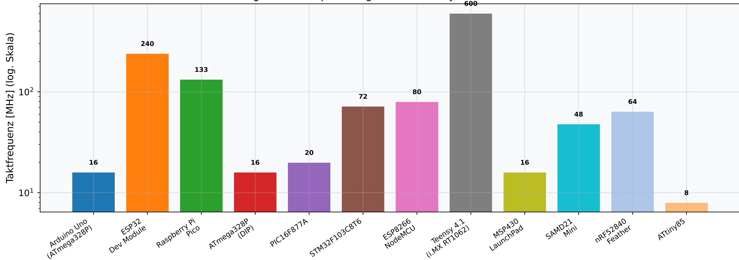
Abbildung 1 - Taktfrequenzvergleich aller analysierten Mikrocontroller
