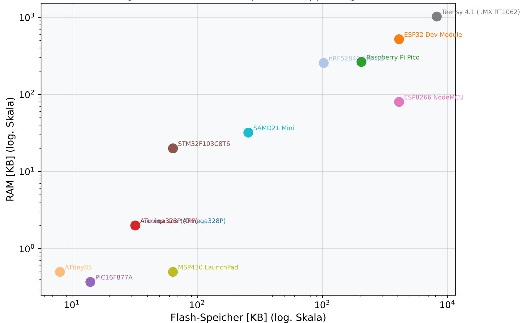
Abbildung 2 – Flash- vs. RAM-Kapazität (doppelt-logarithmisch)
