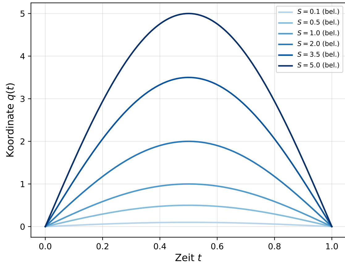
Klassisch: kontinuierliches Wirkungsspektrum
