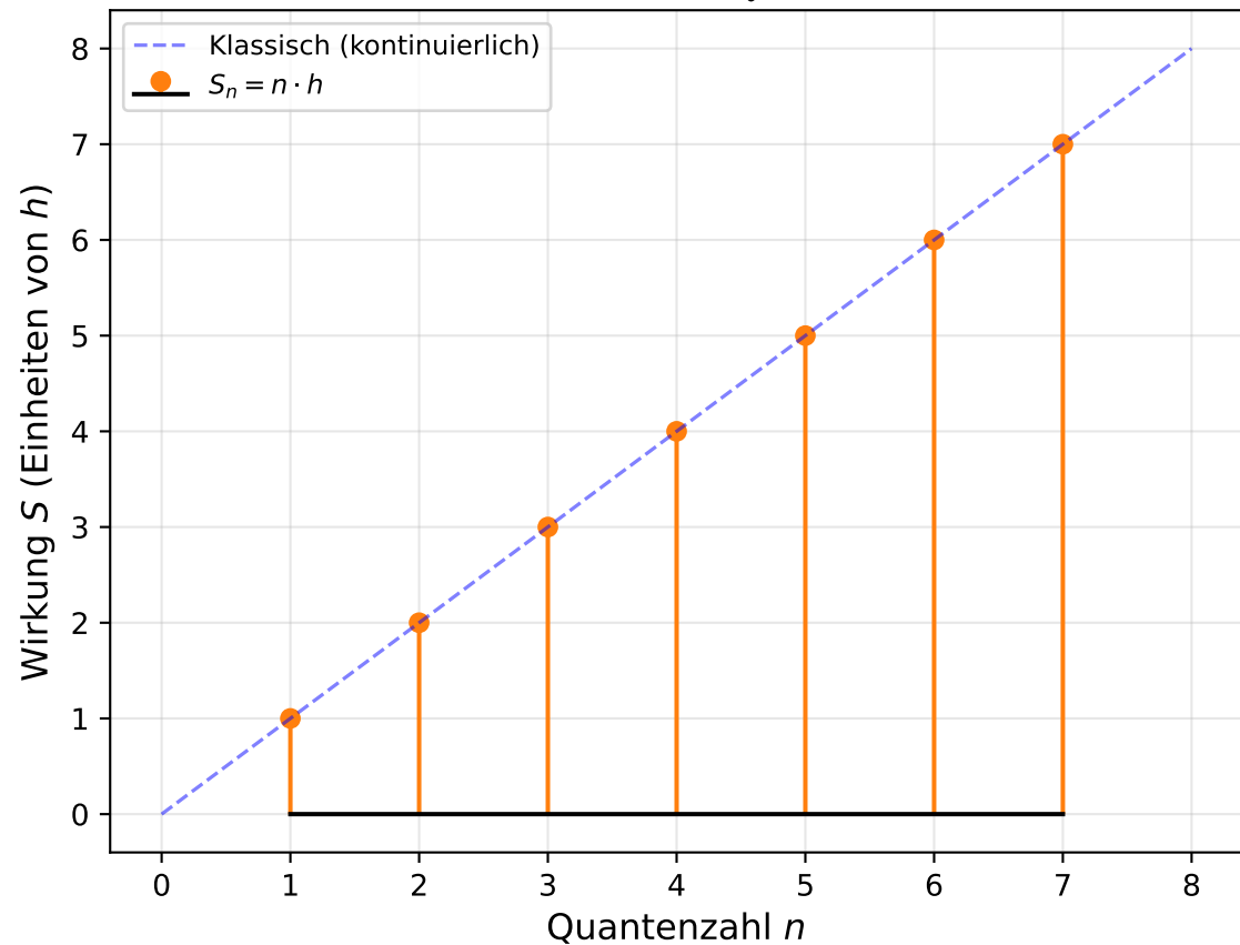
Bohr-Sommerfeld: \oint p dq = nh
