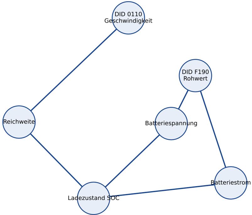
Signal-Abhängigkeitsgraph G_S
