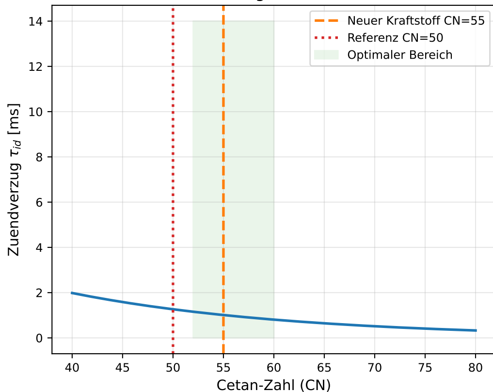
Zuendverzög vs. Cetan-Zahl
