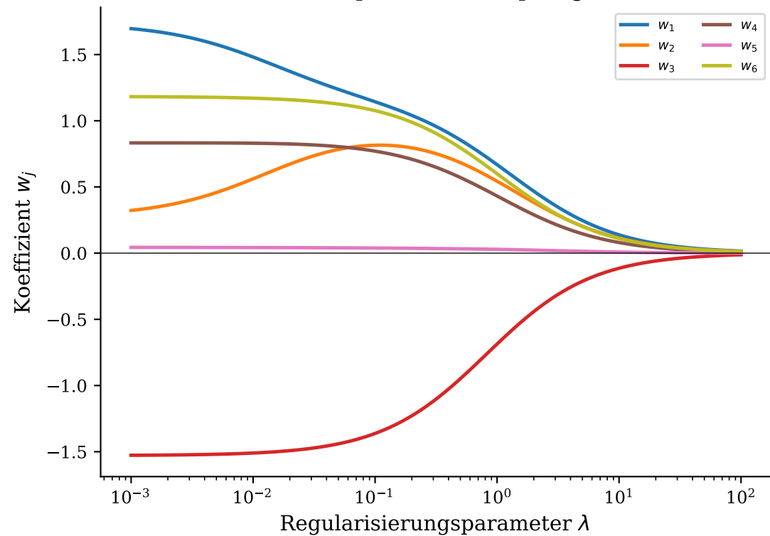
Ridge-Regularisierungspfad (L2-Depensions-Dämpfung)
