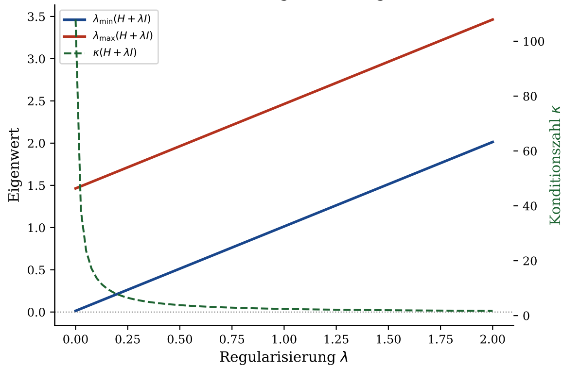
Klassen-Übergang DP-IV \rightarrow DP-I durch L2-Regularisierung
