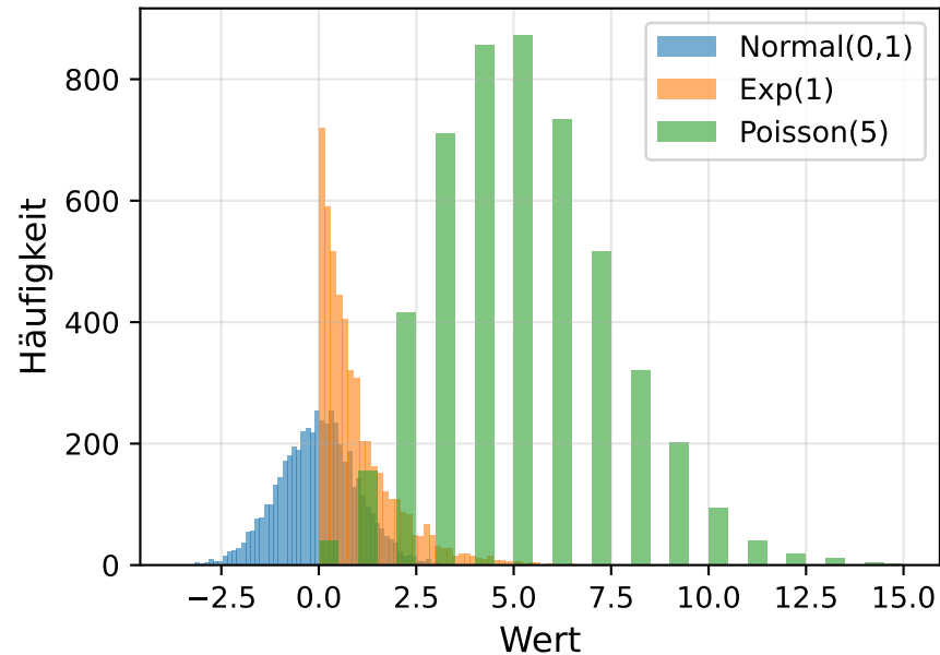
Zufallsverteilungen (NumPy)
