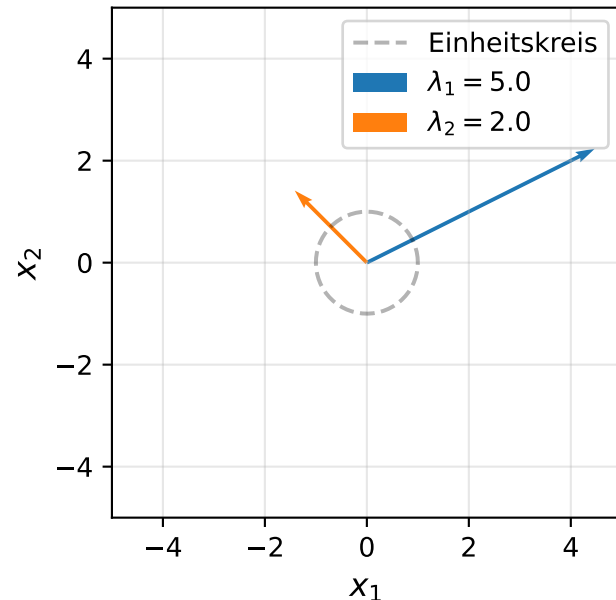
Eigenvektoren / Eigenwerte
