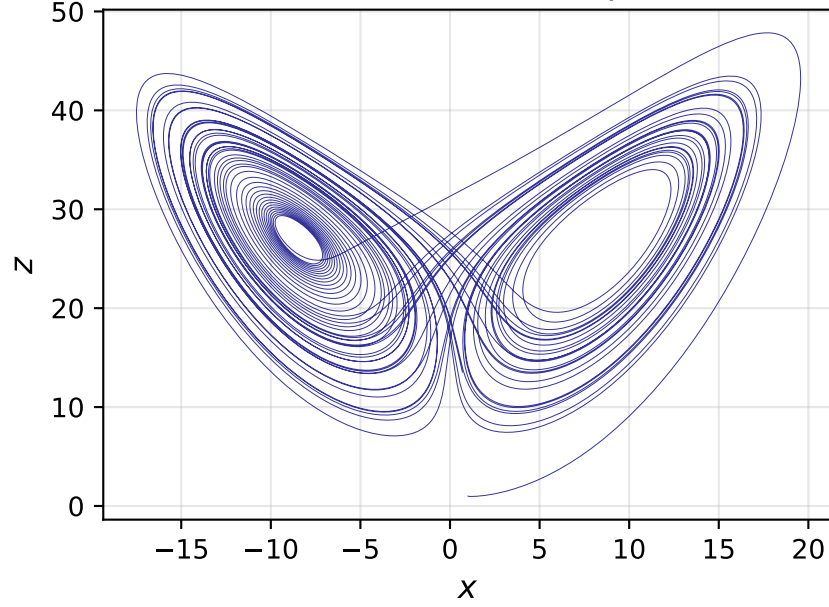
Lorenz-Attraktor (xz-Projektion)
