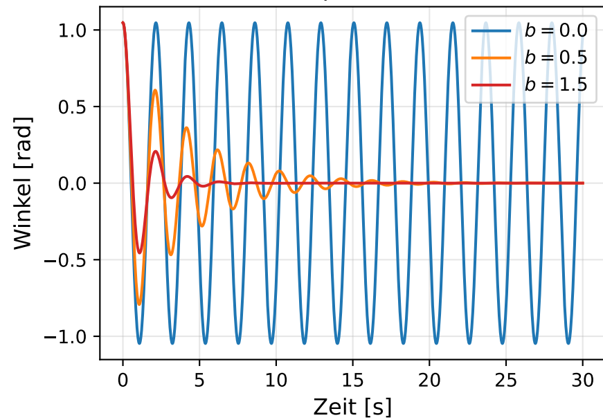
Gedämpftes Pendel
