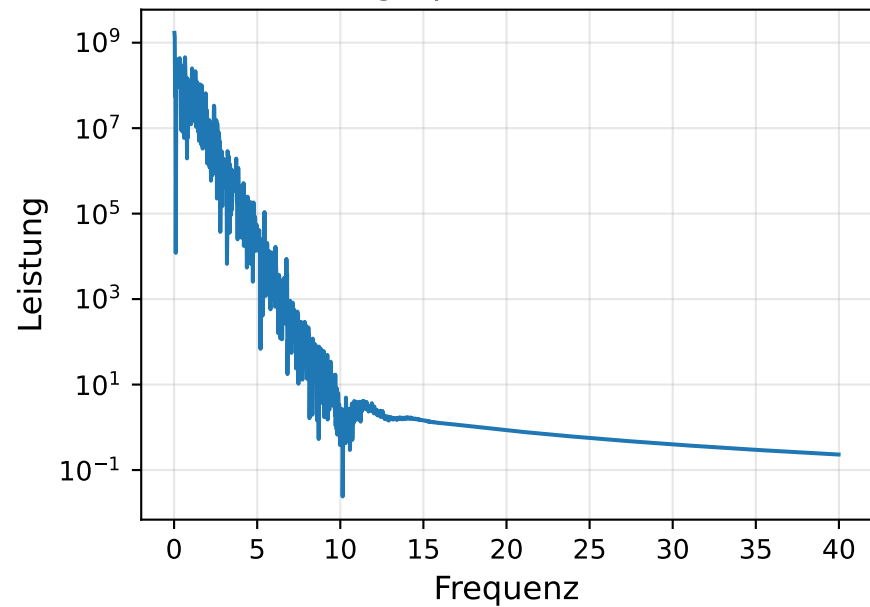
Leistungsspektrum (Lorenz x)
