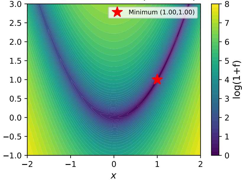
Rosenbrock-Funktion (L-BFGS-B)
