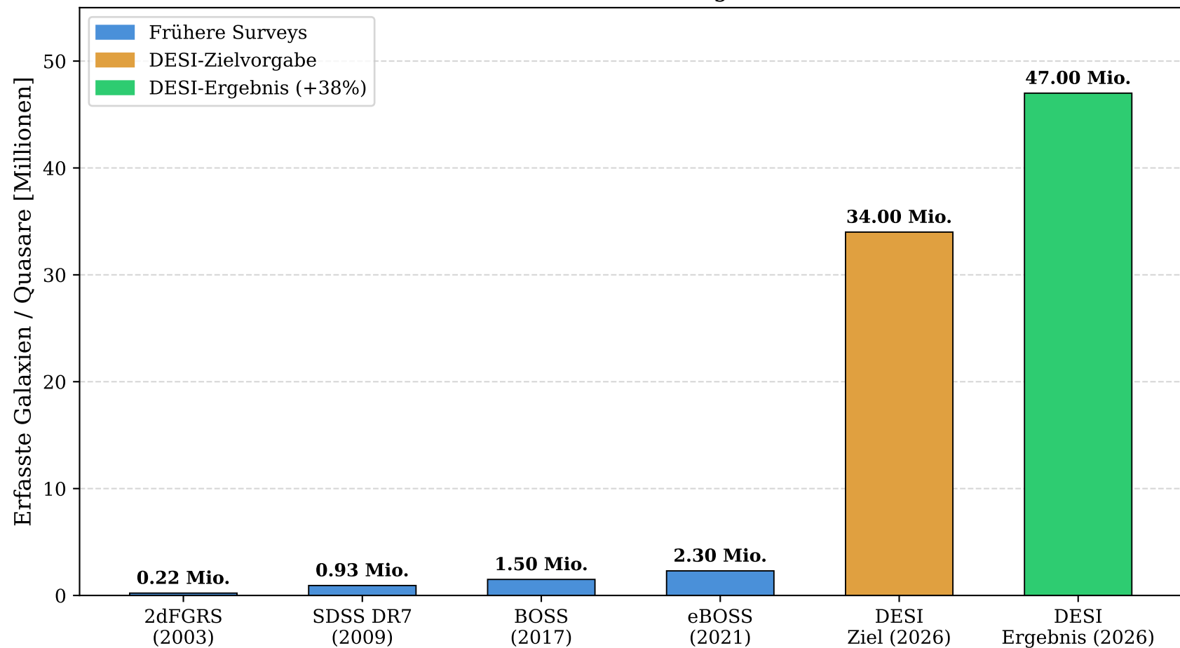
Abbildung 1: Galaxienerfassung großer spektroskopischer Surveys im historischen Vergleich
