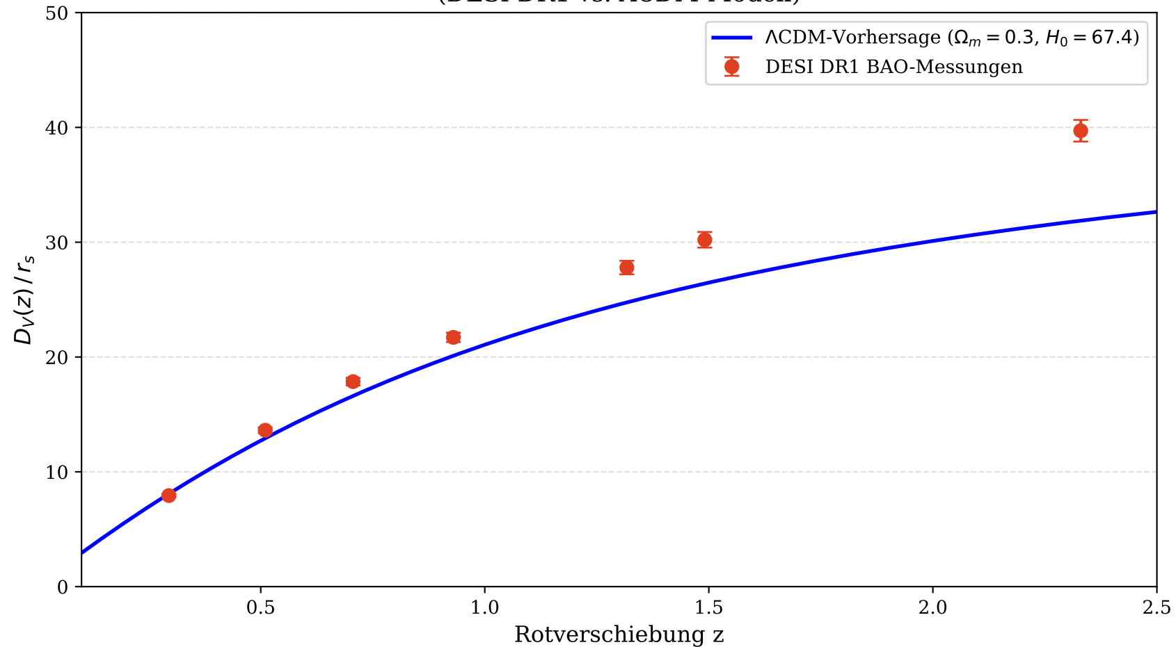
Abbildung 3: BAO-Skalenlänge als Funktion der Rotverschiebung (DESI DR1 vs. \Lambda CDM-Modell)
