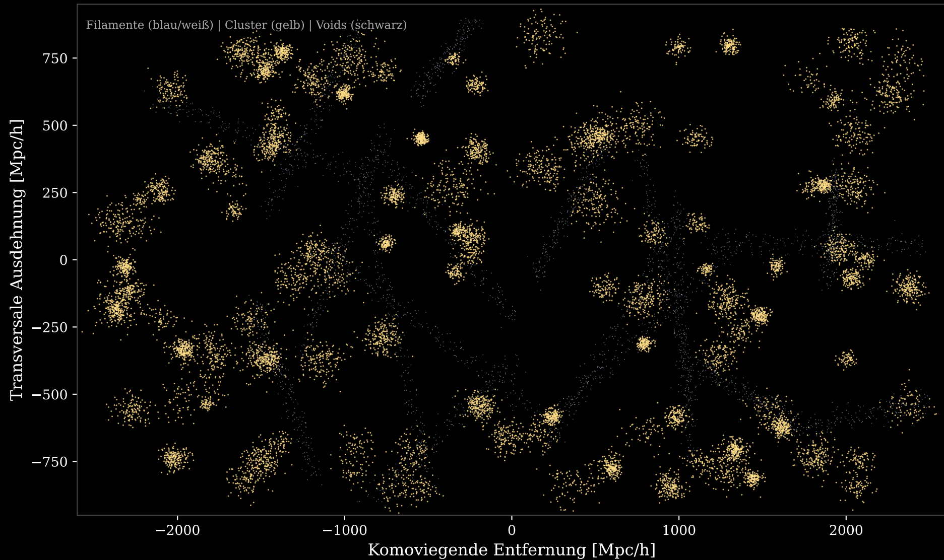
Abbildung 5: Modellerte großräumige Struktur (kosmisches Netz) - DESI-inspirierter Galaxien-Slice bei z \approx 0.5
