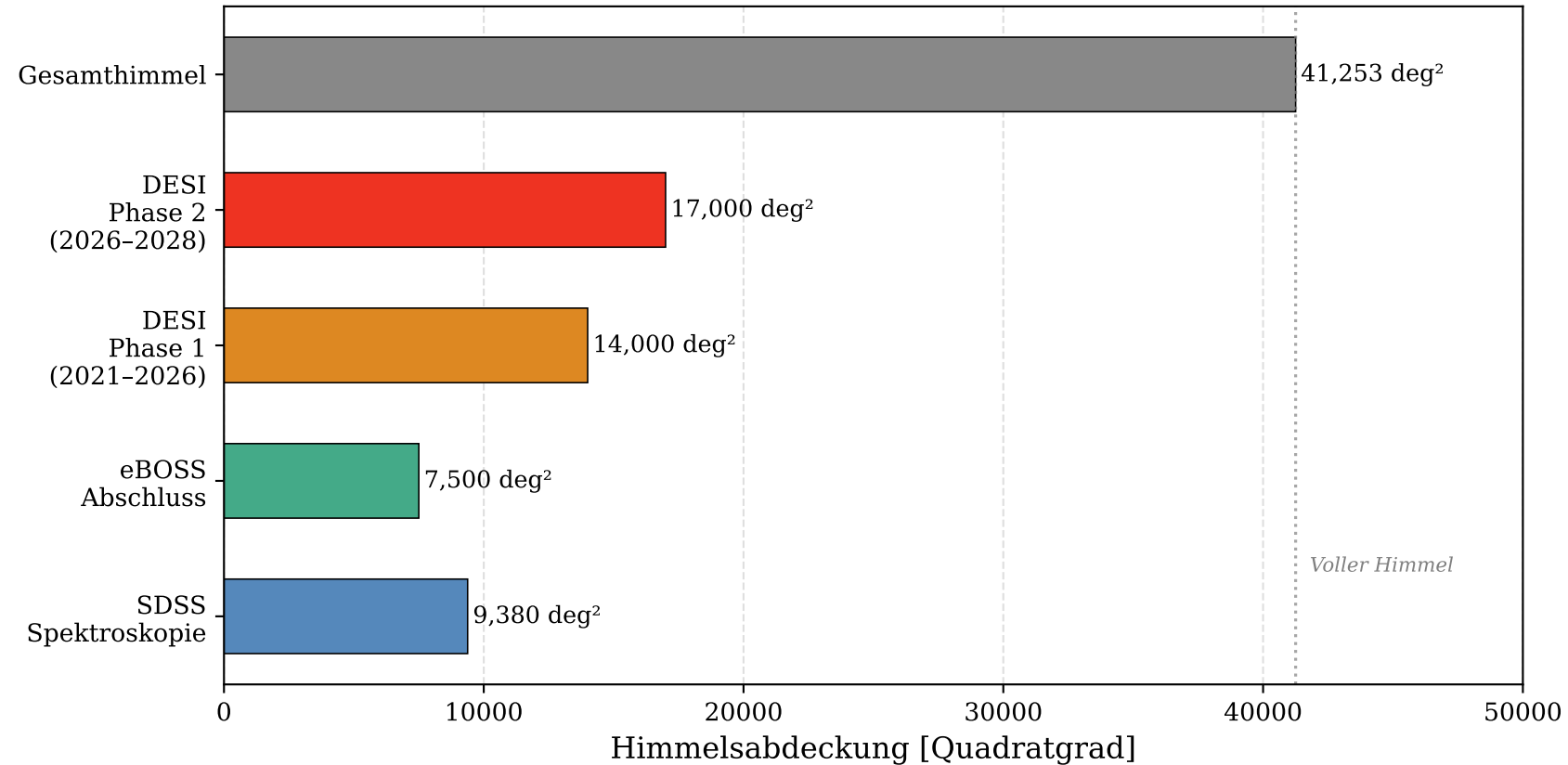
Abbildung 6: Himmelsabdeckung spektroskopischer Surveys (DESI Phase 1 vs. Phase 2 Ausdehnung)
