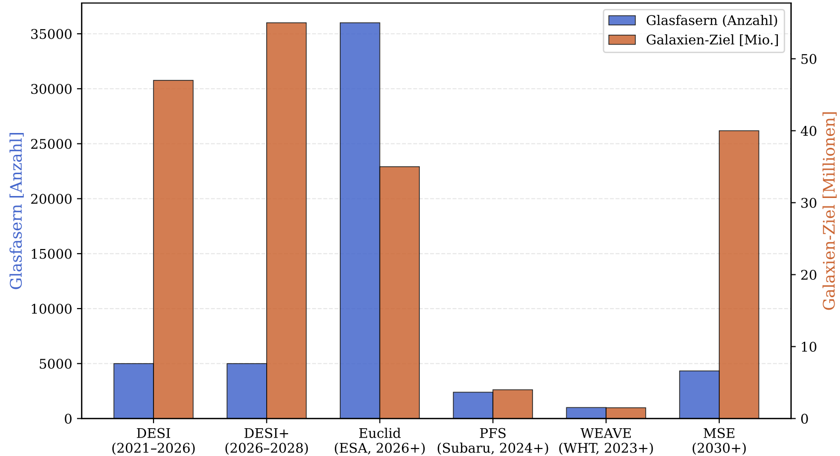
Abbildung 8: Leistungsvergleich aktueller und zukünftiger spektroskopischer Surveying-Instrumente
