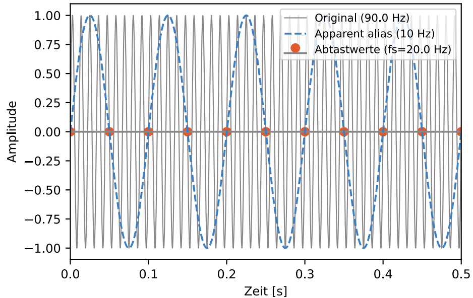
Aliasing: 90.0 Hz bei f_s=20.0 Hz \rightarrow 10.0 Hz
