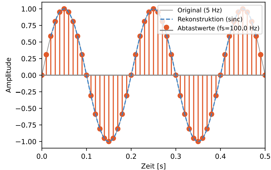
Perfekte Rekonstruktion ( f_0=5.0 Hz, f_s=100.0 Hz)
