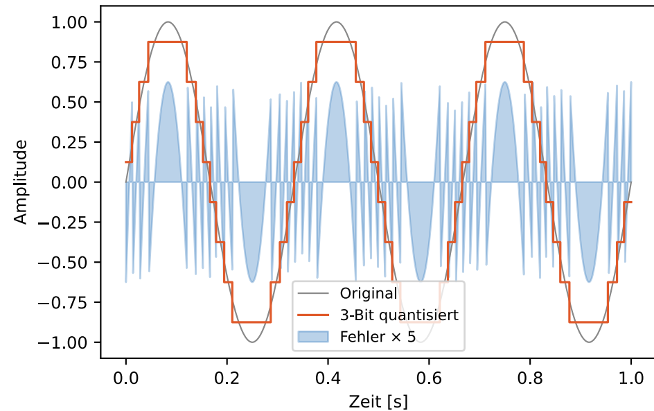
3-Bit Quantisierung (×5 Fehler)
