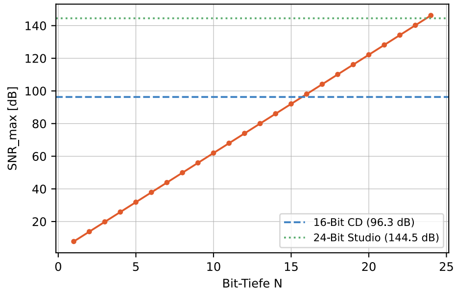
Theoretisches SNR: 6.02 \cdot N + 1.76 dB
