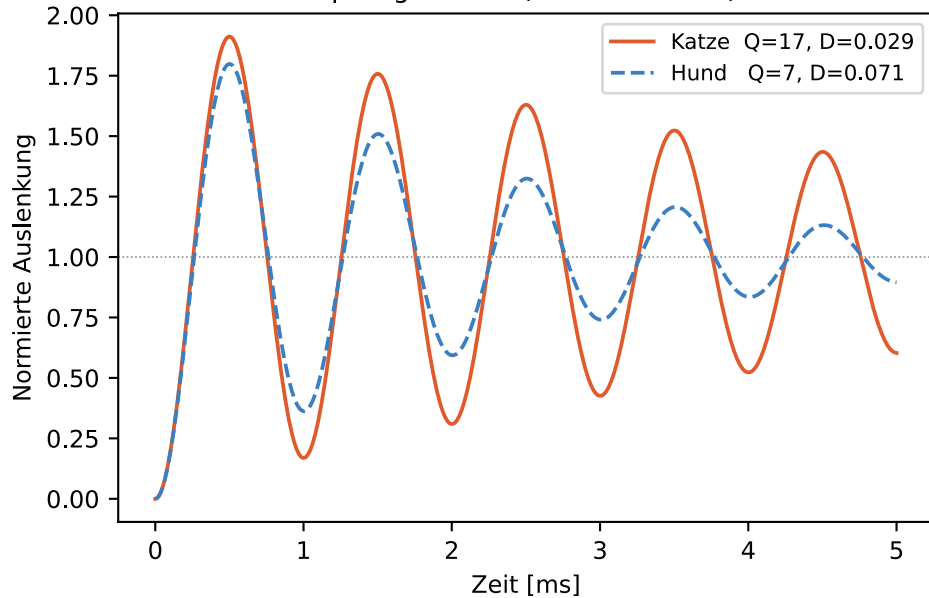
Sprungantwort ( f_0 = 1000.0 Hz)
