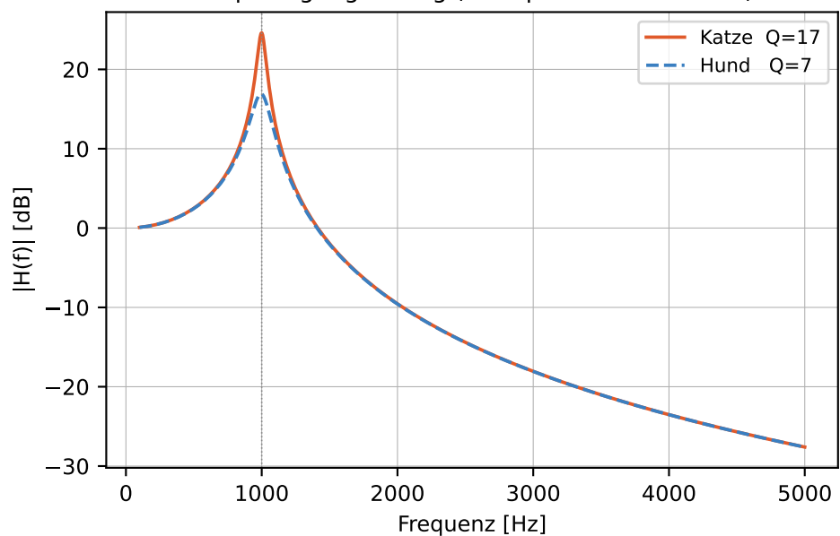
Frequenzgang-Betrag (Bandpasscharakteristik)
