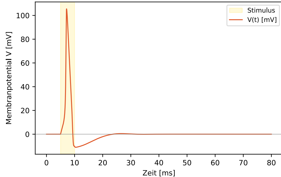
Aktionspotential (HH 1952, I=10\text{ }\mu\text{A}/\text{cm}^2 )
