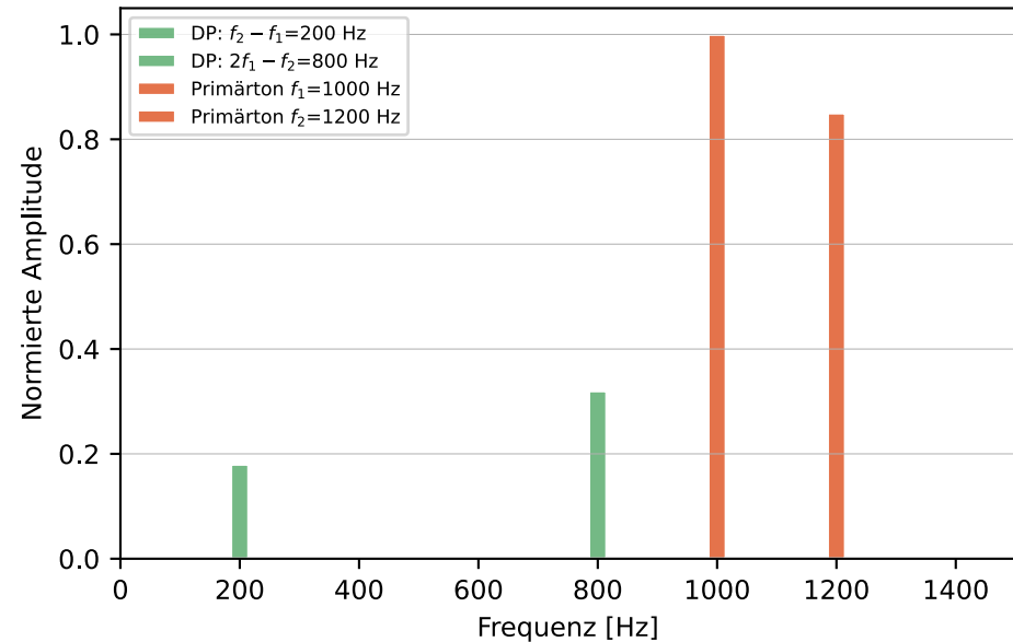
Zwei-Ton-Verzerrungsprodukte
