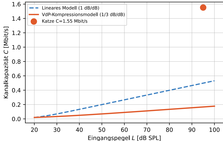
Shannon-Kapazität: linear vs. nichtlinear
