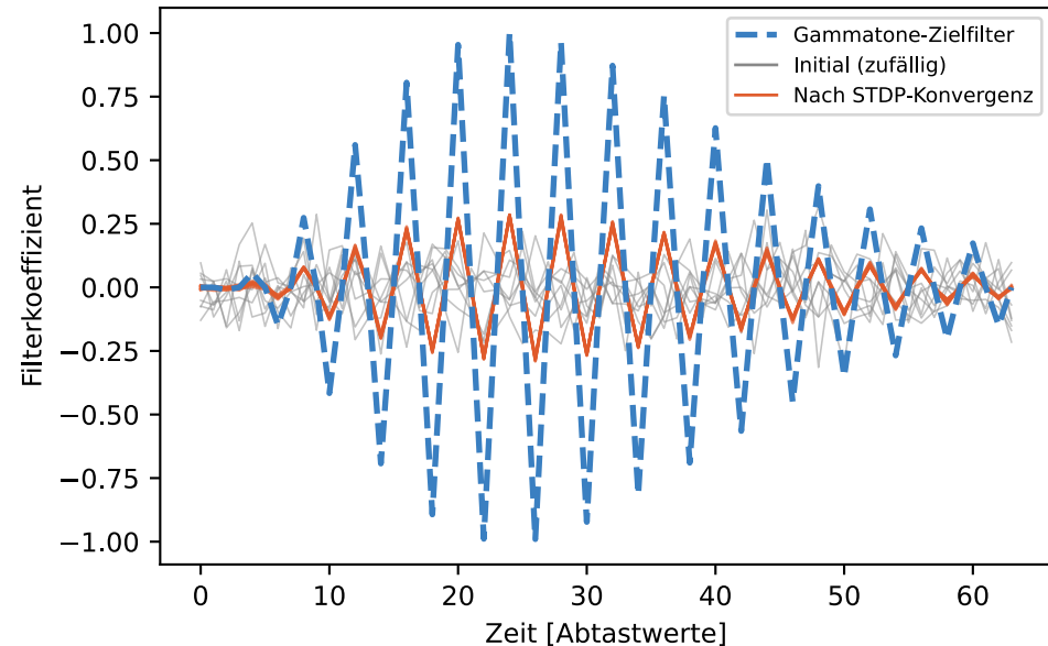
STDP-Selbstorganisation: zufällig → Gammatone
