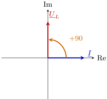
Spule
