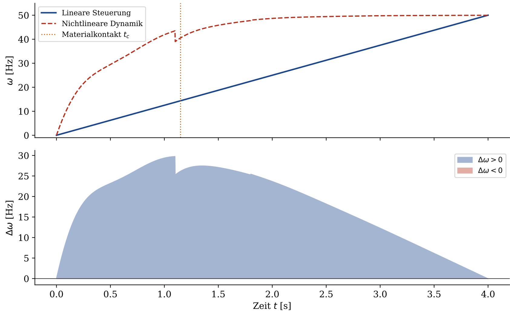
Abbildung 1 - Winkelgeschwindigkeit \omega(t) beim Sägeblatt-Anlauf
