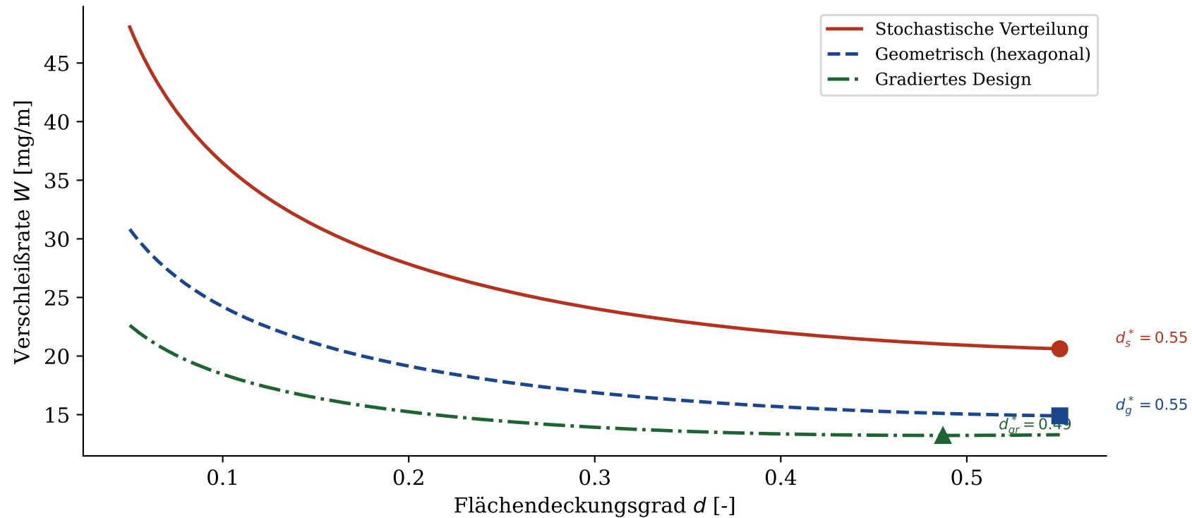
Abbildung 4 – Verschleißrate W(d) in Abhängigkeit des Diamant-Flächendeckungsgrads
