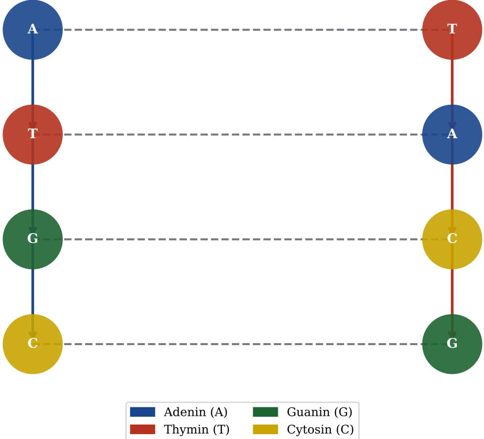
Graph-Repräsentation G_{DNA} (Knoten = Basen, Kanten = Bindungen)
