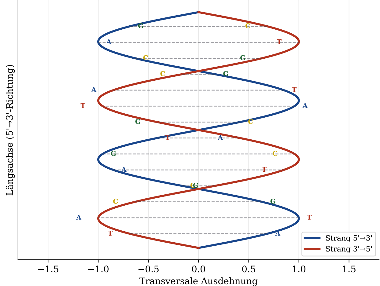
DNA-Doppelhelix mit komplementären Basenpaaren
