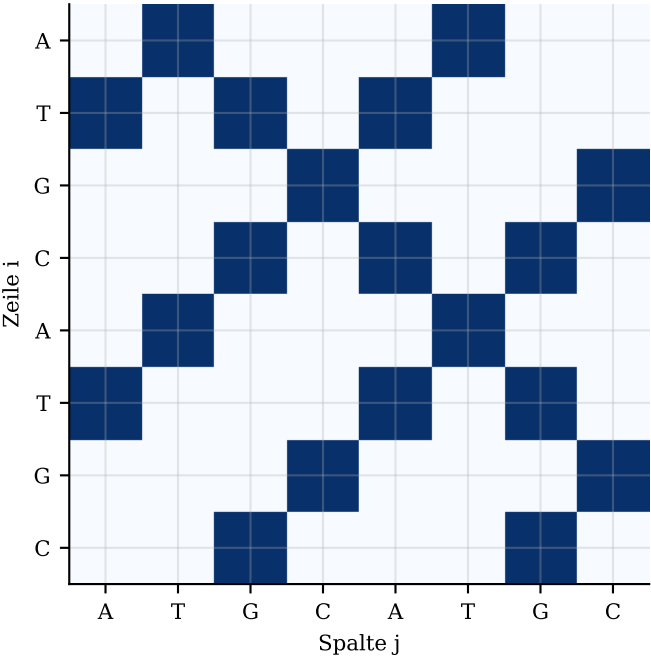
Referenz: ATGCATGC
