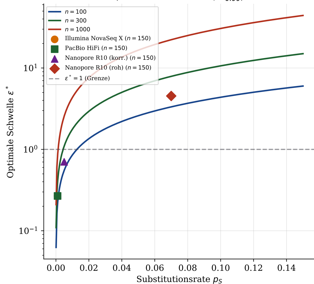
Abb. 22 - Optimale Schwellwahl \varepsilon^* nach Sequenziertechnologie Optimale Schwelle \varepsilon^* vs. Fehlerrate (nur Substitutionen, z_{0.99} )
