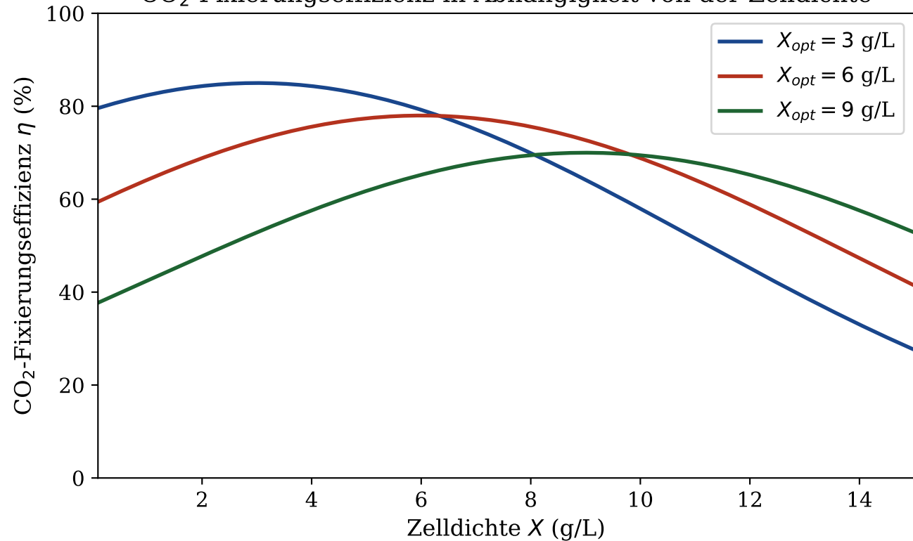
CO 2 -Fixierungseffizienz in Abhängigkeit von der Zelldichte
