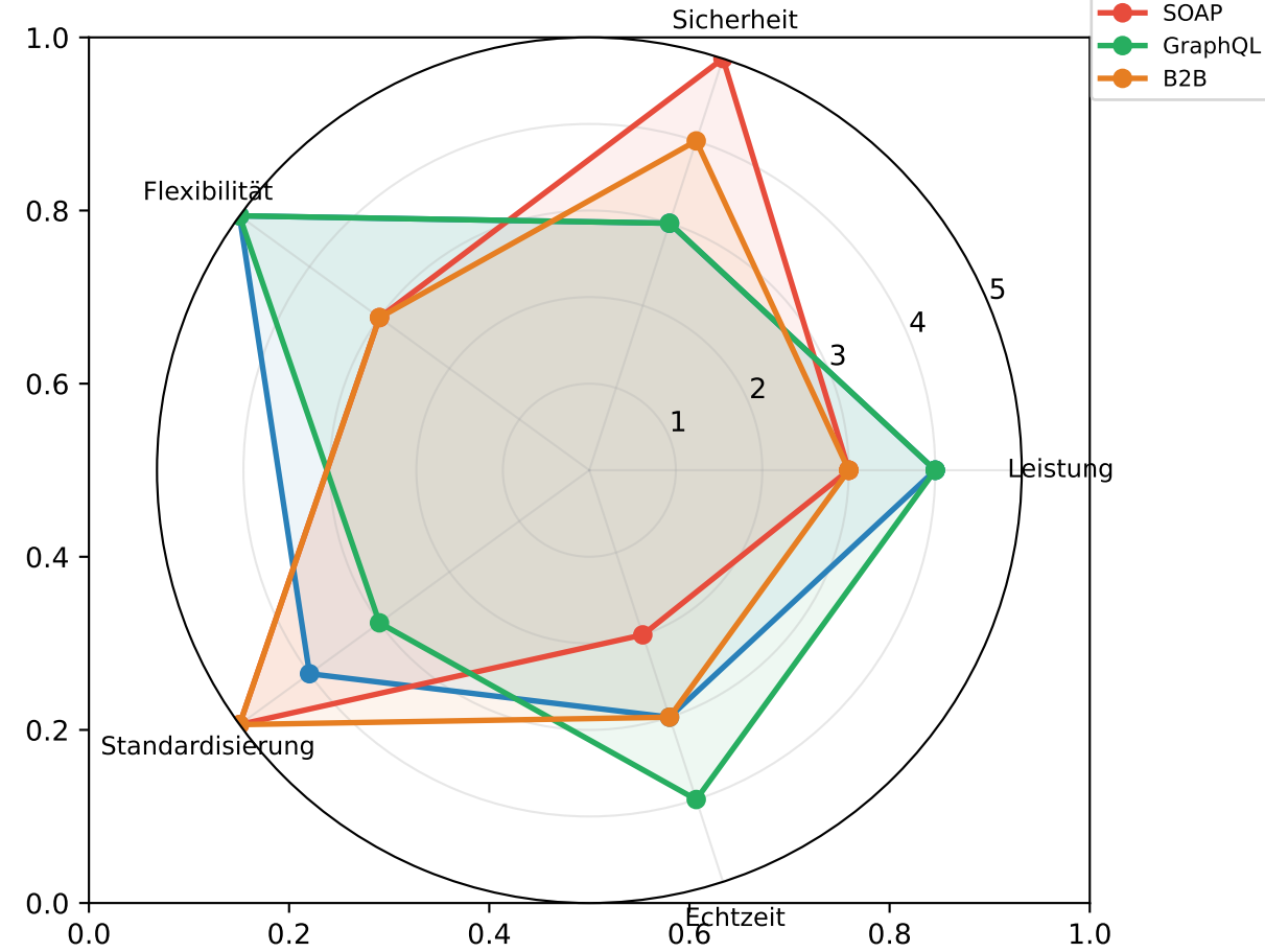
API-Eigenschaftsprofil (Radar)
