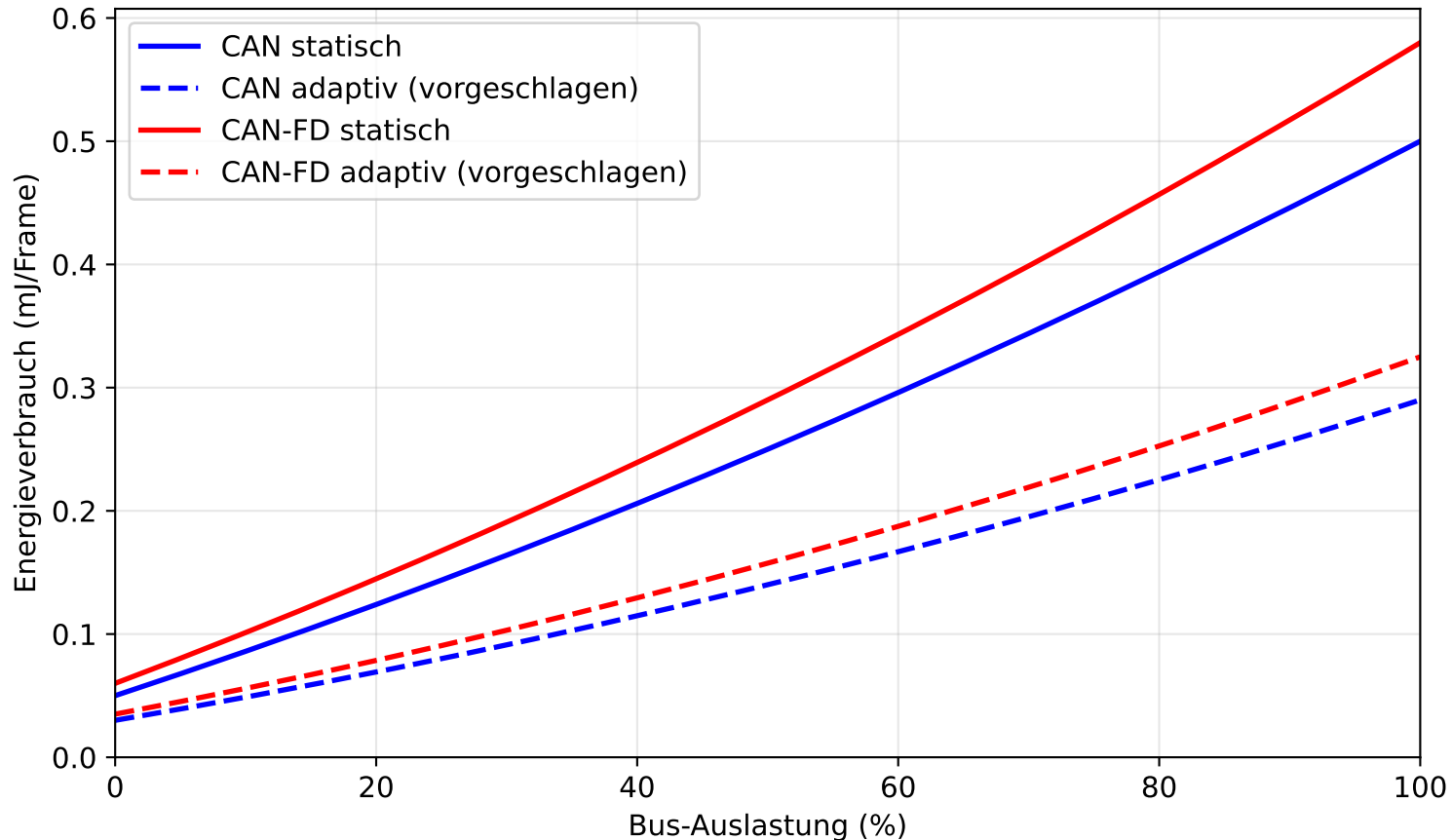
Energieverbrauch in Abhängigkeit der Bus-Auslastung
