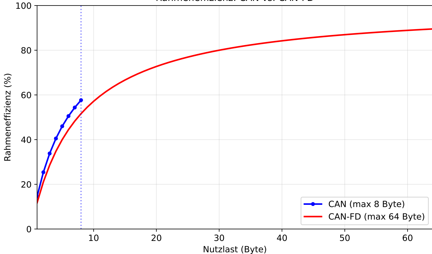
Rahmeneffizienz: CAN vs. CAN-FD
