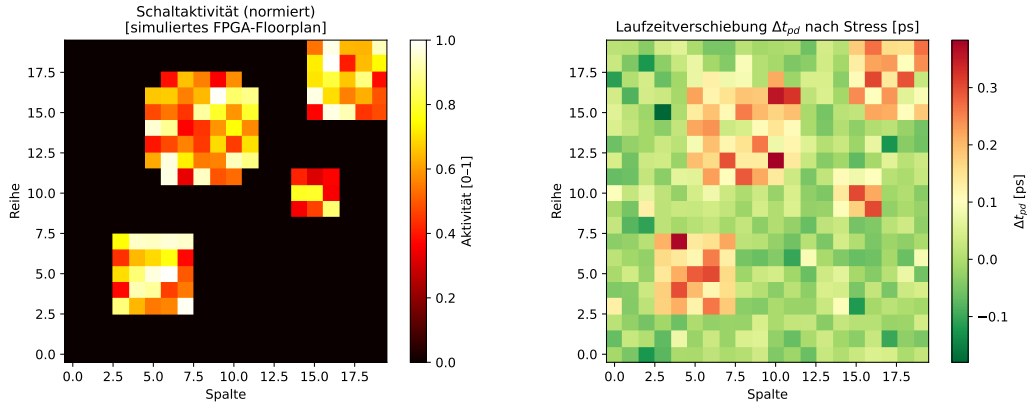
Abbildung 6: Pfadverifikation durch Timing-Shift-Heatmap: Links die simulierte Schaltaktivität auf einem 20 \times 20 -Tile-FPGA-Floorplan (normiert auf 0–1). Rechts die resultierende Laufzeitverschiebung \Delta t_{pd} nach Stresstest. Die räumliche Korrelation beider Karten ermöglicht die Identifikation aktiver Pfade.
