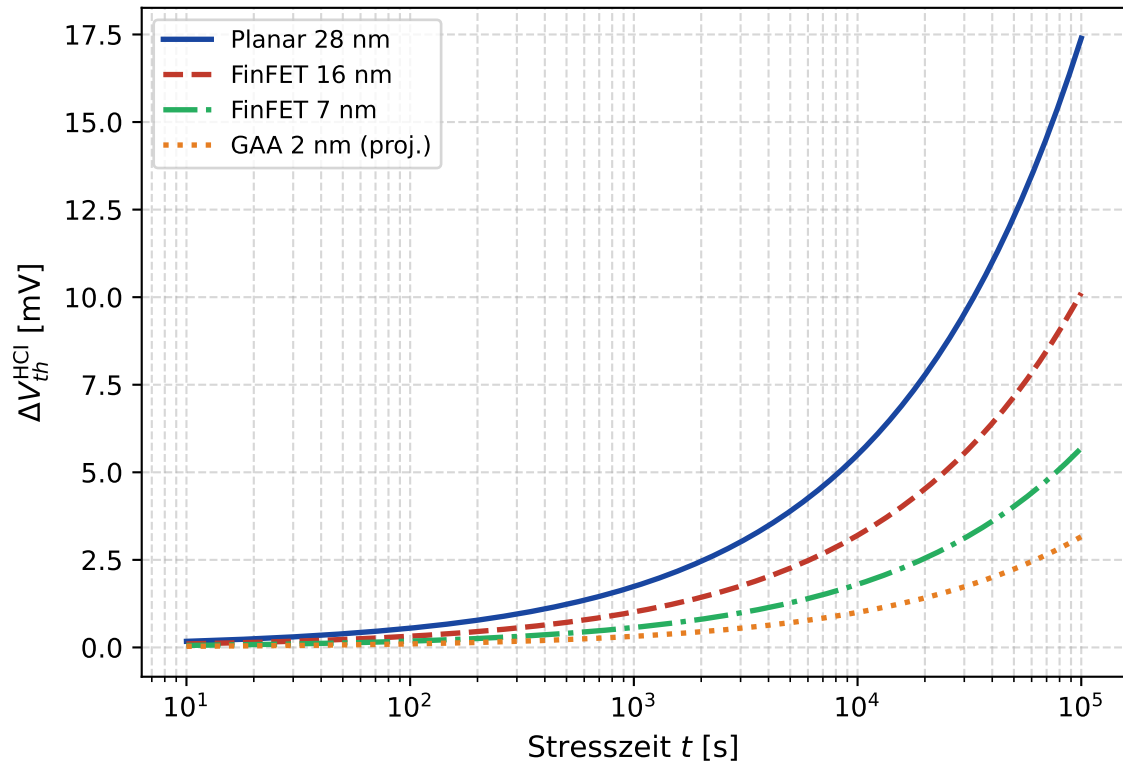
HCl: Planar vs. FinFET vs. GAA
